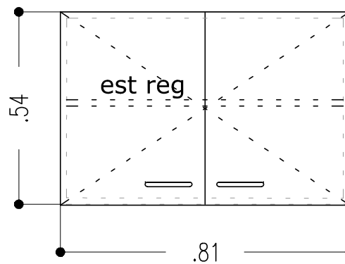
M6 - MODULO DOS PUERTAS ALACENA cantidad: 2
