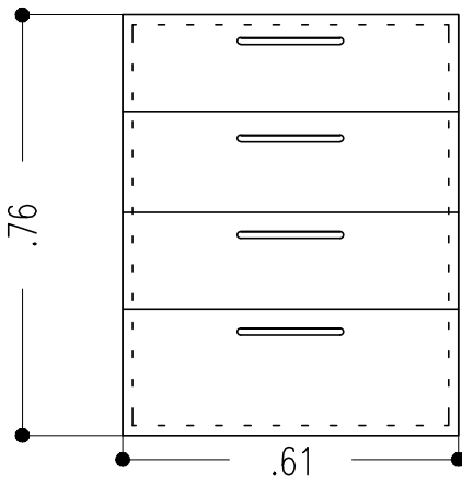
M3 - MESADA DE MELAMINA cantidad: 1 tabla de doble placa de 18mm e: 36mm
